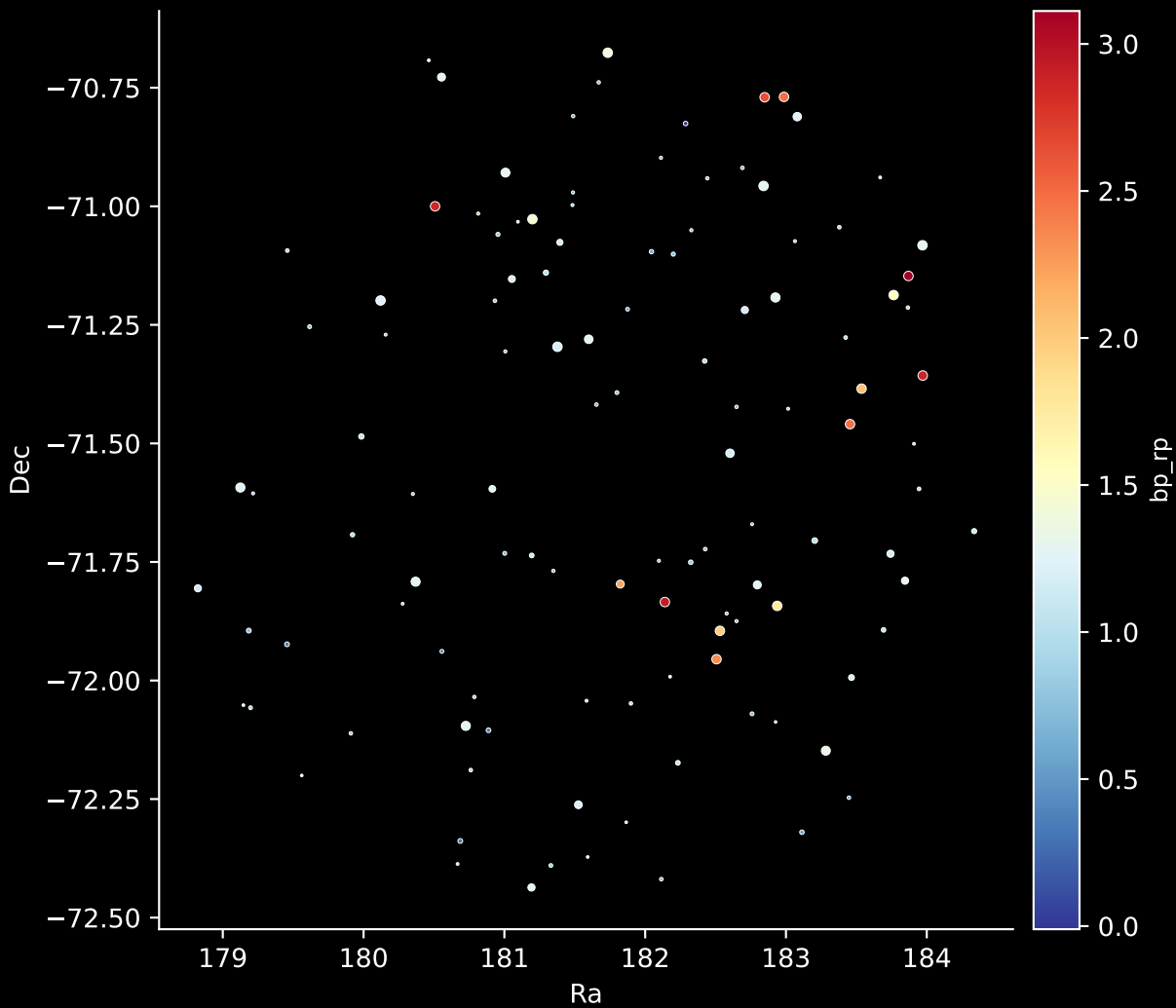
APOGEE DR17 Field: [282-32-O_TESS] Stars: 115
