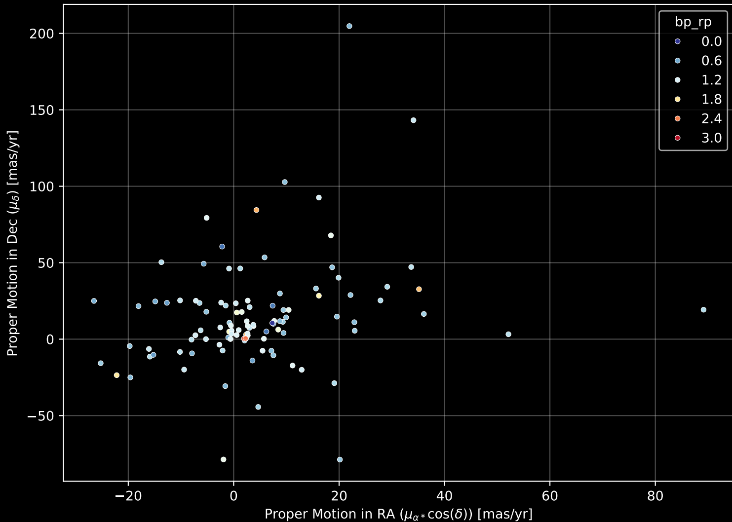
APOGEE DR17 Field: [282-32-O_TESS] Proper Motion Diagram (n= 115)
