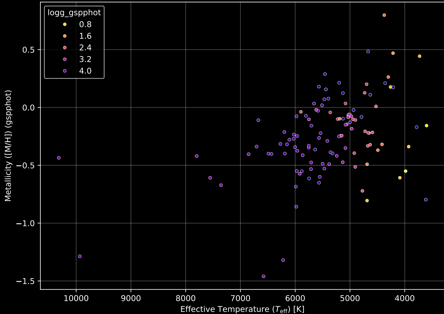
APOGEE DR17 Field: [282-32-O_TESS] Stellar Population Parameters (n= 115)
