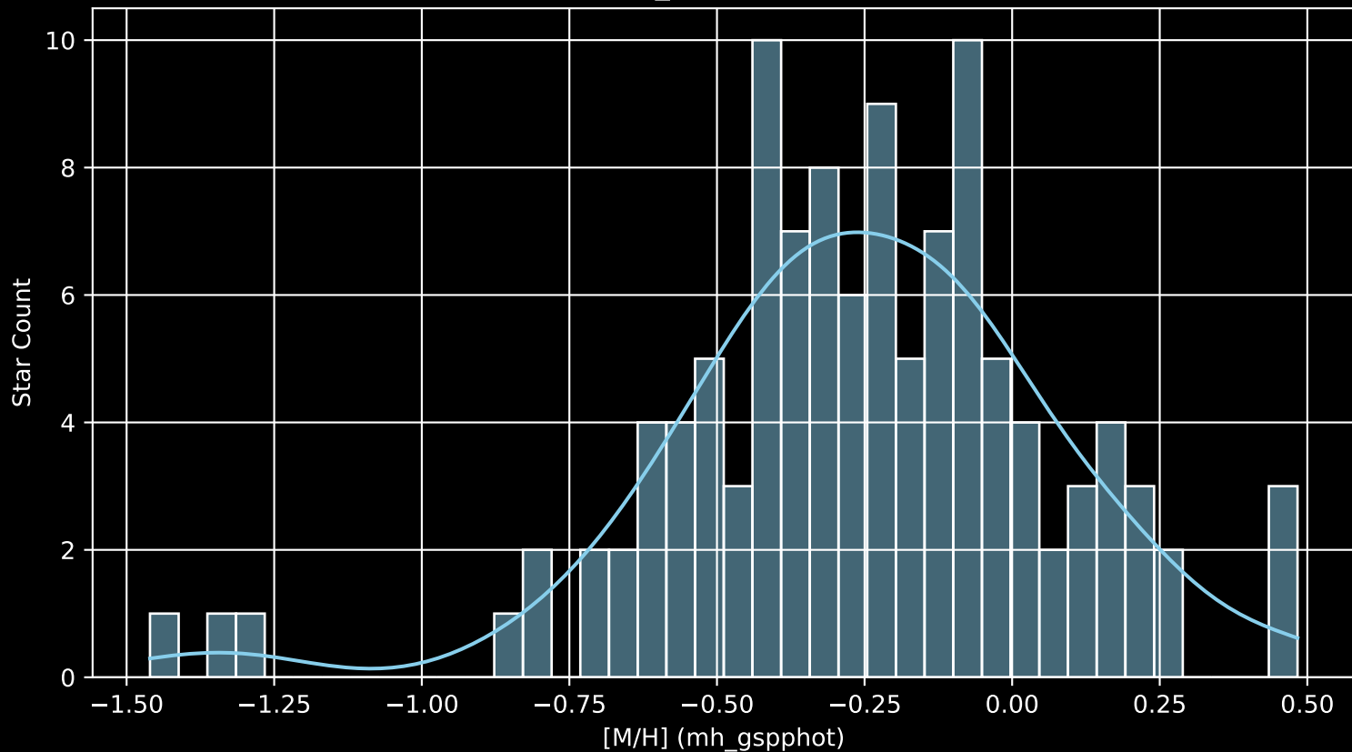
APOGEE DR17 Field: [282-32-O_TESS [M/H] (mh_gspphot) (n= 114)
